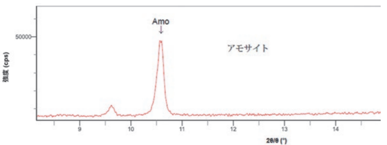
■ X線回折定量分析例(アスベスト標準の定量X線チャート)
